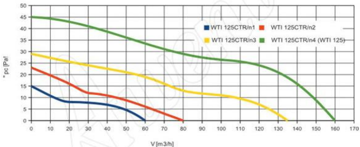
ГРАФИКА НА ВЕНТИЛАТОР Ф125 С 4-РИ СКОРОСТИ АКО ВЕНТИЛАТОРЪТ Е ОБИКНОВЕН ДА СЕ ГЛЕДА ЗЕЛЕНАТА ГРАФИКА.
